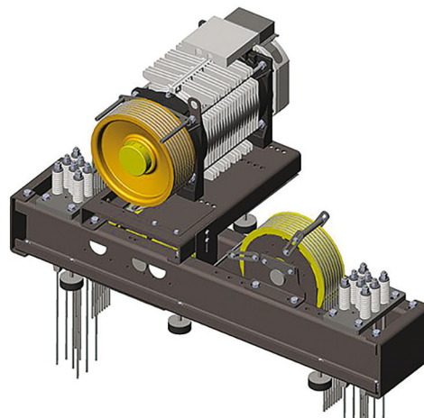
Fot. 6 Wyciągarka MRL, nowoczesne urządzenie windowe, które łączy dużą moc z małymi wymiarami. Global Lift
